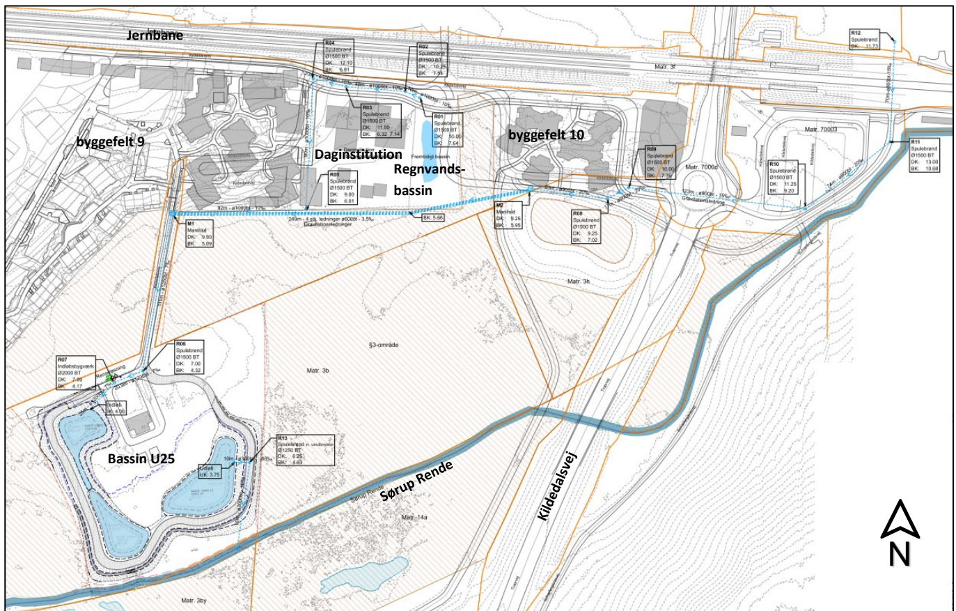
Figur 14 Tracé - Forslag 2 (se tegning KB_K10_H1_LP_BAU25)
