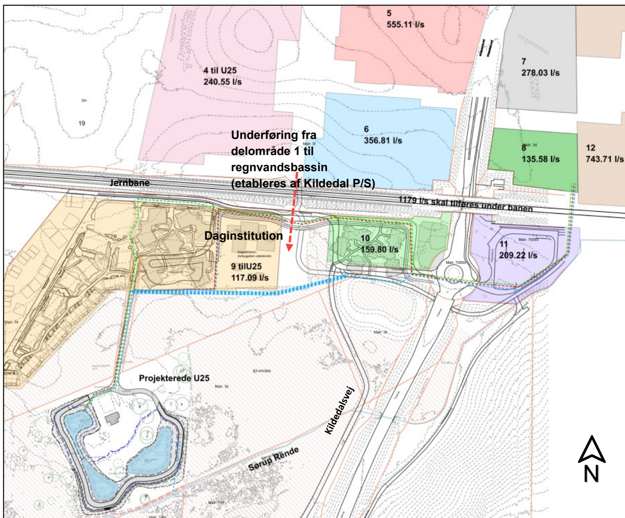
Figur 11 Oversigtskort med byggefelter (markeret med farver og numre)
