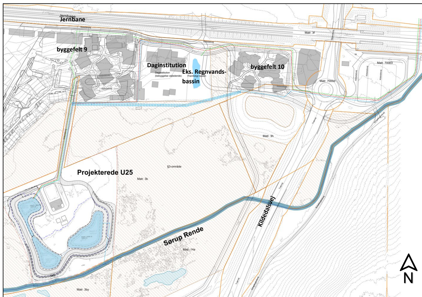
Figur 12: Screenede ledningstraceer til regnvandsledningen. Forslag 1 = grøn linje, Forslag 2 = blå linje, Forslag 3 = rød linje (Se yderligere beskrivelse for forslag 1 og 3 i bilag 6)
