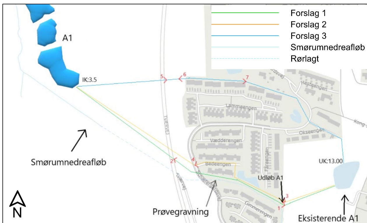
Figur 10 Oversigtskort for mulige ledningstracéer mellem det eksisterende og det projekterede Bassin A1, opmålt trace for rørlagt vandløb samt pile for markering af billedokumentation. Billede nr. 1 se Figur 13 , billede nr. 2 se Figur 14,- mens der for billede nr. 3 til 7 henviser til figurer i Bilag 6.
