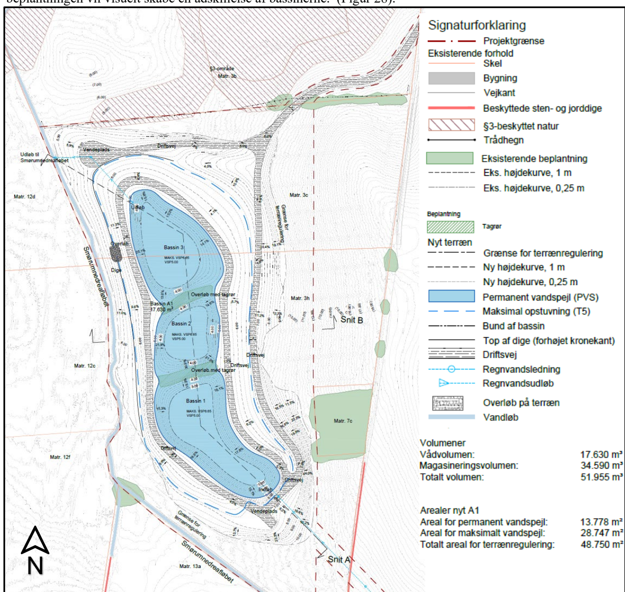
Figur 28 Det projekterede Bassin A1 udformes som tre våde bassiner med et fælles forsinkelsesvolumen og adgangsvveje. Se tegning KB_K02_H1_SP_BAA1
