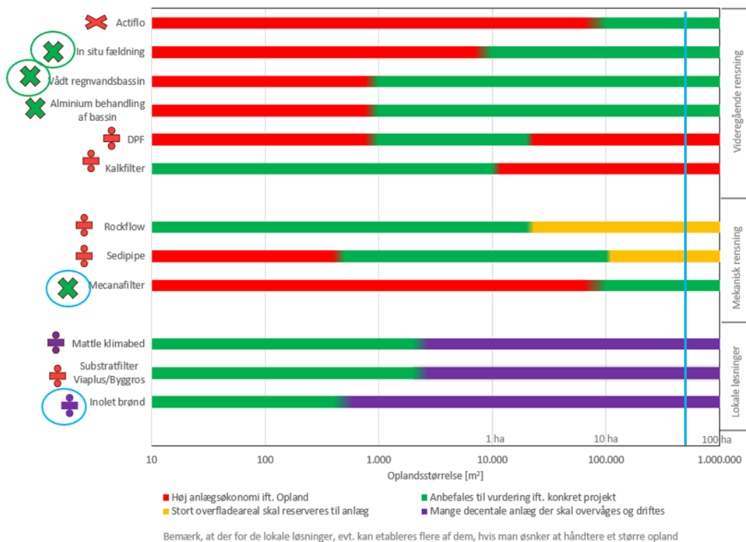
Figur 20 Skema for valg af videregående rensning på Bassin A1 med et opland på ca. 70 ha red (blå lodret linje). X med en grøn ring udpeger den primære rens metode mens blå ring udpeger løsninger som der senere kan suppleres med hvis den primære rensstrategi ikke er tilstrækkelig effektiv.
