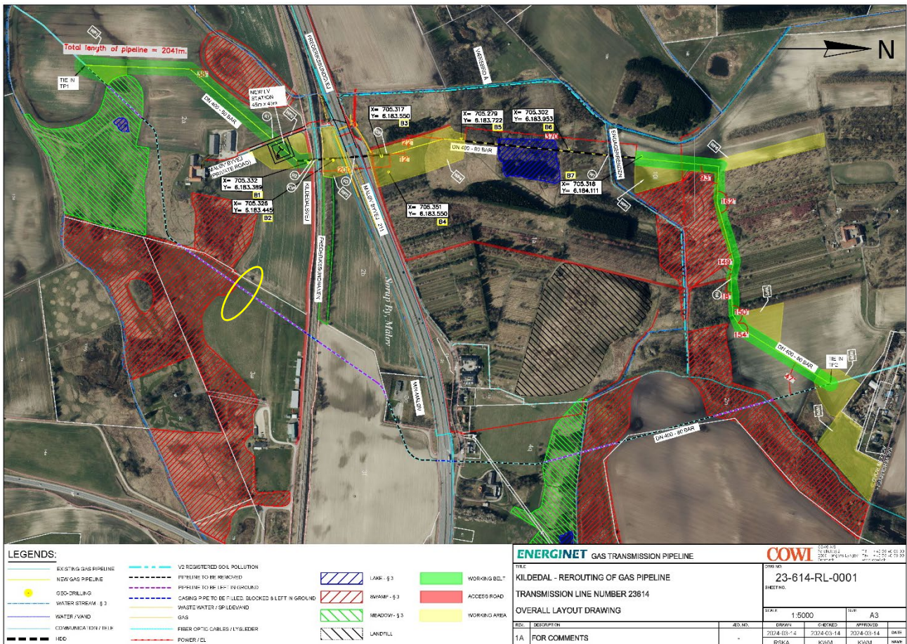
Figur 1. Gasledningens kommende tracé (gul linje, underboring med sort-gul-stiplet), nuværende placering er vist med sort/lilla linje. Ved gul oval efterlades ledningen IKKE, da der ca. her skal etableres et regnvandsbassin, som kræver at ledningen fjernes.
