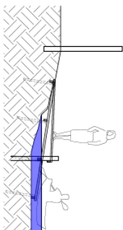
Tværsnit A-A
